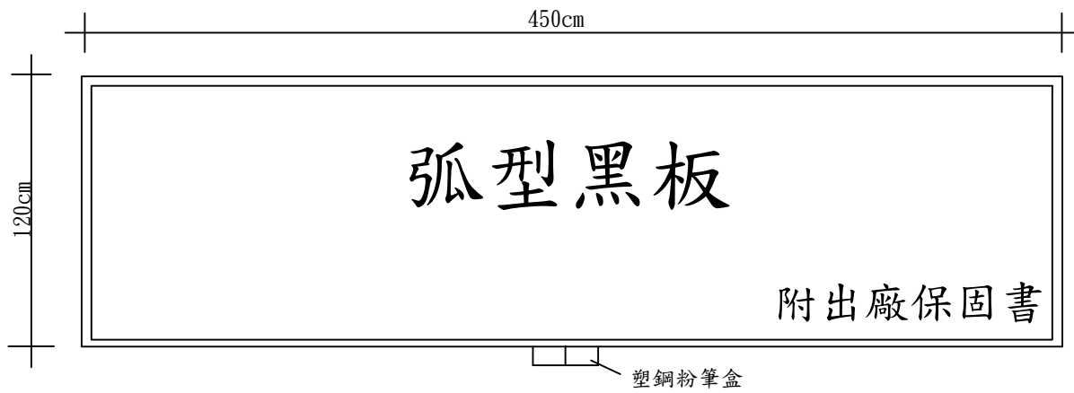
正面圖
